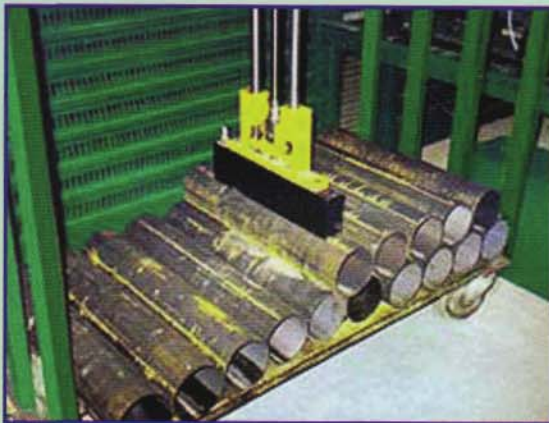
Descargador electromagnético
